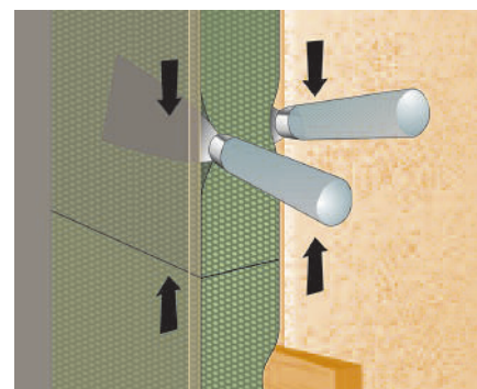
Afbeelding 2: Stuik aansluiting verticale voegen
